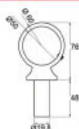
ΣΤΗΡΙΓΜΑ ΚΟΥΠΑΣΤΗΣ Φ50 ΣΕ ΚΟΛΩΝΑ Φ40 PILLAR CONNECTION 40x50
