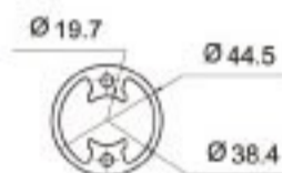
ΕΝΩΤΙΚΟ ΓΩΝΙΑΣ ΜΑΣΙΦ Φ50 (ΕΣΩΤΕΡΙΚΟ) BEND CONNECTION Φ50 (INTERNAL)
