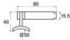
ΣΤΗΡΙΞΗ ΚΟΥΠΑΣΤΗΣ Φ50 ΡΥΘΜΙΖΟΜΕΝΗ ADJUSTABLE "L" CONNECTION
