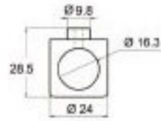
ΣΤΗΡΙΓΜΑ ΜΠΑΡΑΣ Φ16 ΡΥΘΜΙΖΟΜΕΝΟ INTERCONNECTION Φ16
