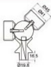
ΓΩΝΙΑ ΡΥΘΜΙΖΟΜΕΝΗ ΓΩΝΙΑΚΗ Φ50 MOTIONAL BEND Φ50 WITH PILLAR CONNECTION
