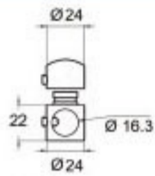
ΣΤΗΡΙΓΜΑ ΜΠΑΡΑΣ Φ16 ΔΙΑΙΡΟΥΜΕΝΟ INTERCONNECTION Φ16 DOUBLE
